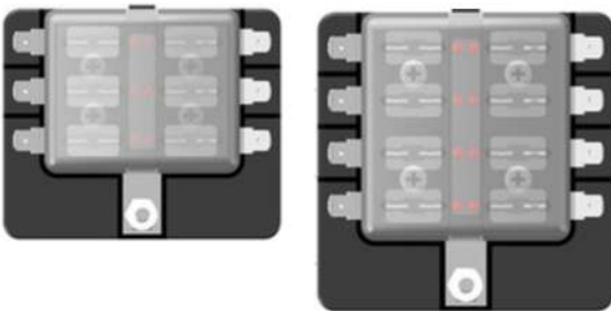
ED0283 Sigorta Kutusu 6'lı İkaz Işıklı Kolay Bağlantı ED0284 Sigorta Kutusu 8'li İkaz Işıklı Kolay Bağlantı
